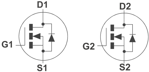
SO8
